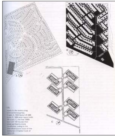
(شكل-2) تنمية اسكانية في هنكاريا بالاستفادة من الطاقة الشمسية. أ- تجميع غير منتظم ب- تجميع متوازي نحو الجنوب. ج- تجميع حول فناء وسطي . المصدر:Roaf,2003,p40
